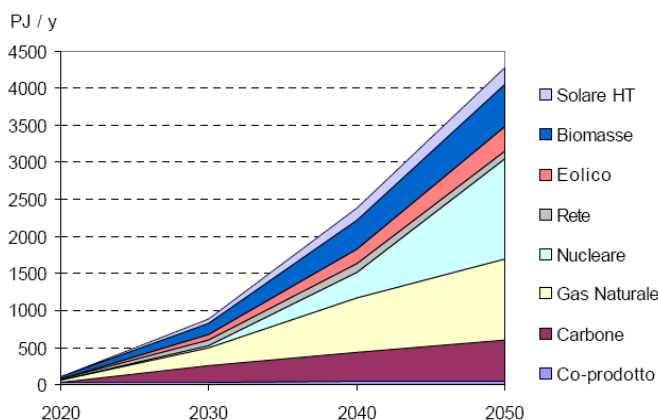
Figura 42 - Mix di produzione dell'idrogeno per i 10 Stati membri dell'UE sulla base delle visioni nazionali
