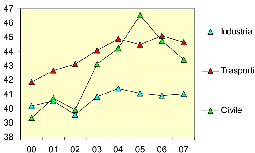
Figura 21 - Consumi di energia per settori di uso finale, trend Italia 2000-2007 (Mtep)
